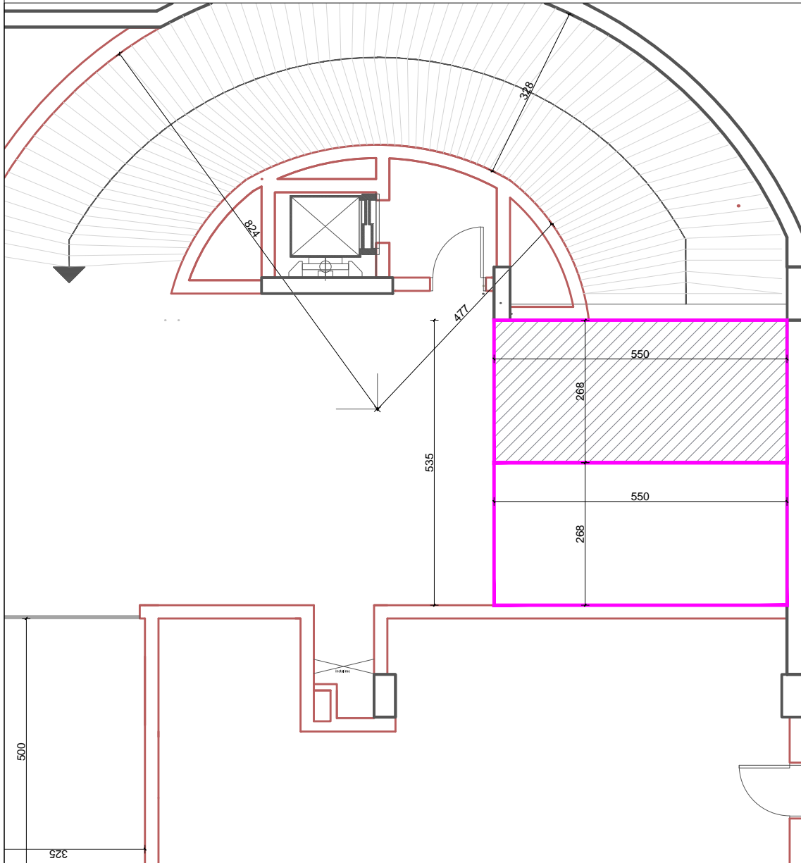
PLANIMETRIA SH 1: 100
