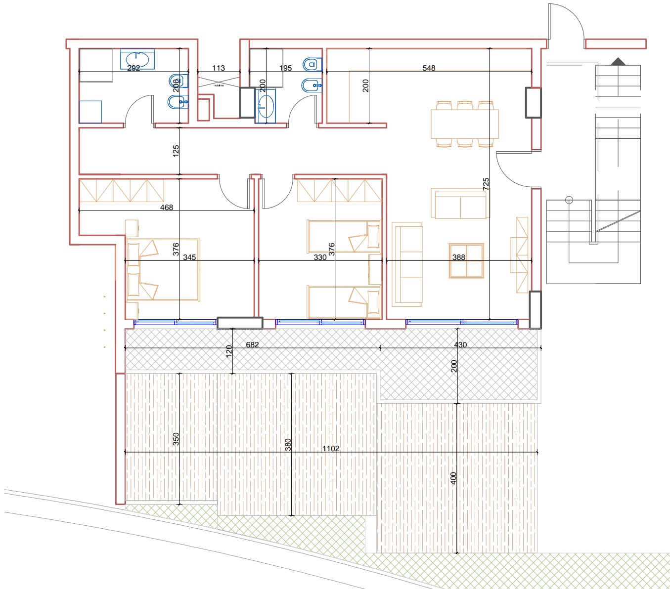
PLANIMETRIA SH 1: 100
