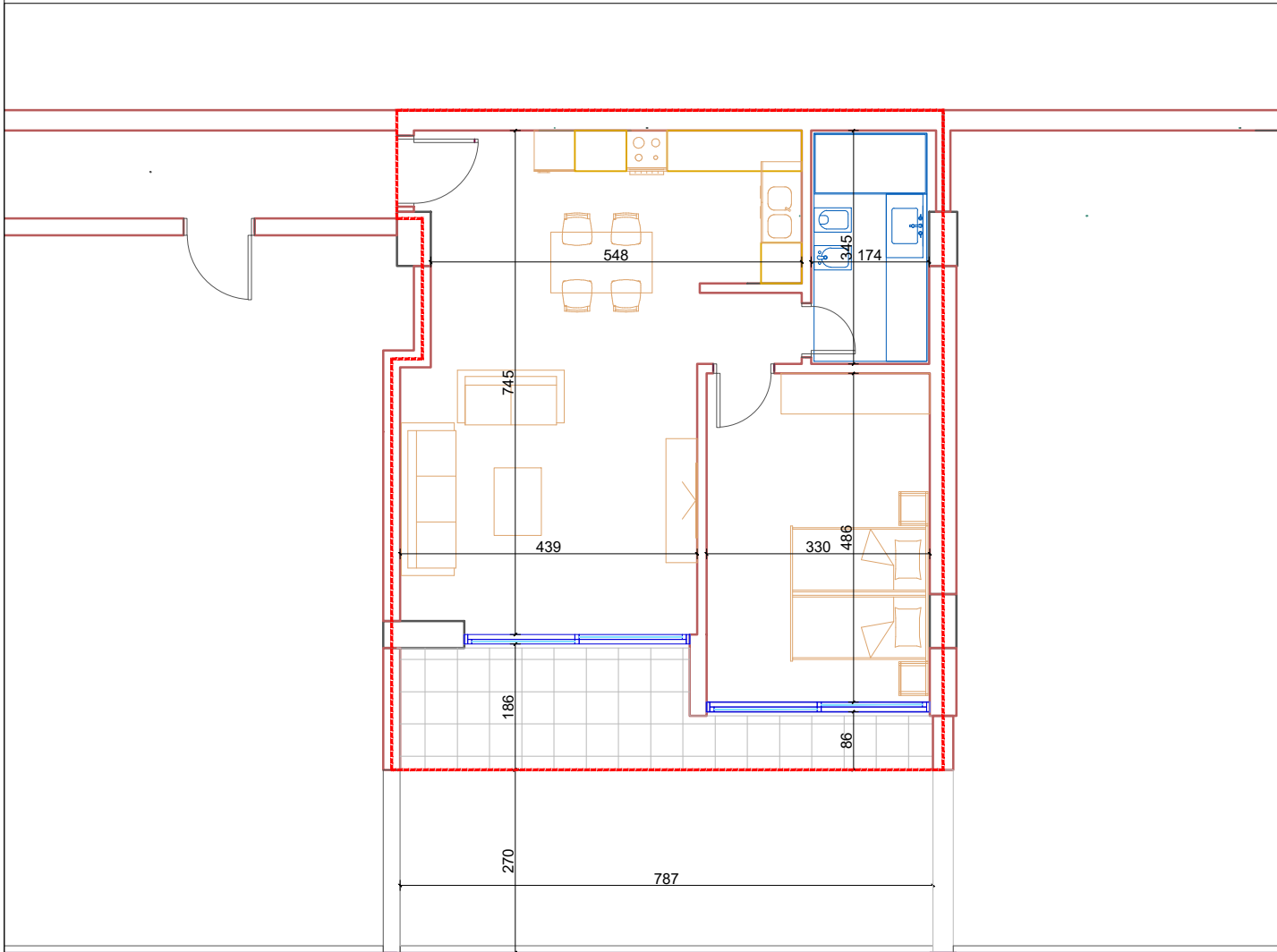
PLANIMETRIA SH 1: 100
