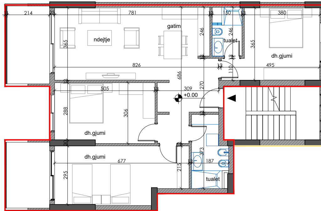
PLANIMETRIA SH 1: 100
