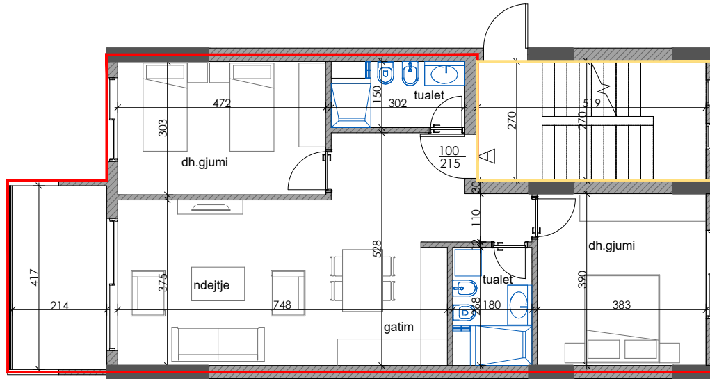
PLANIMETRIA SH 1: 100
