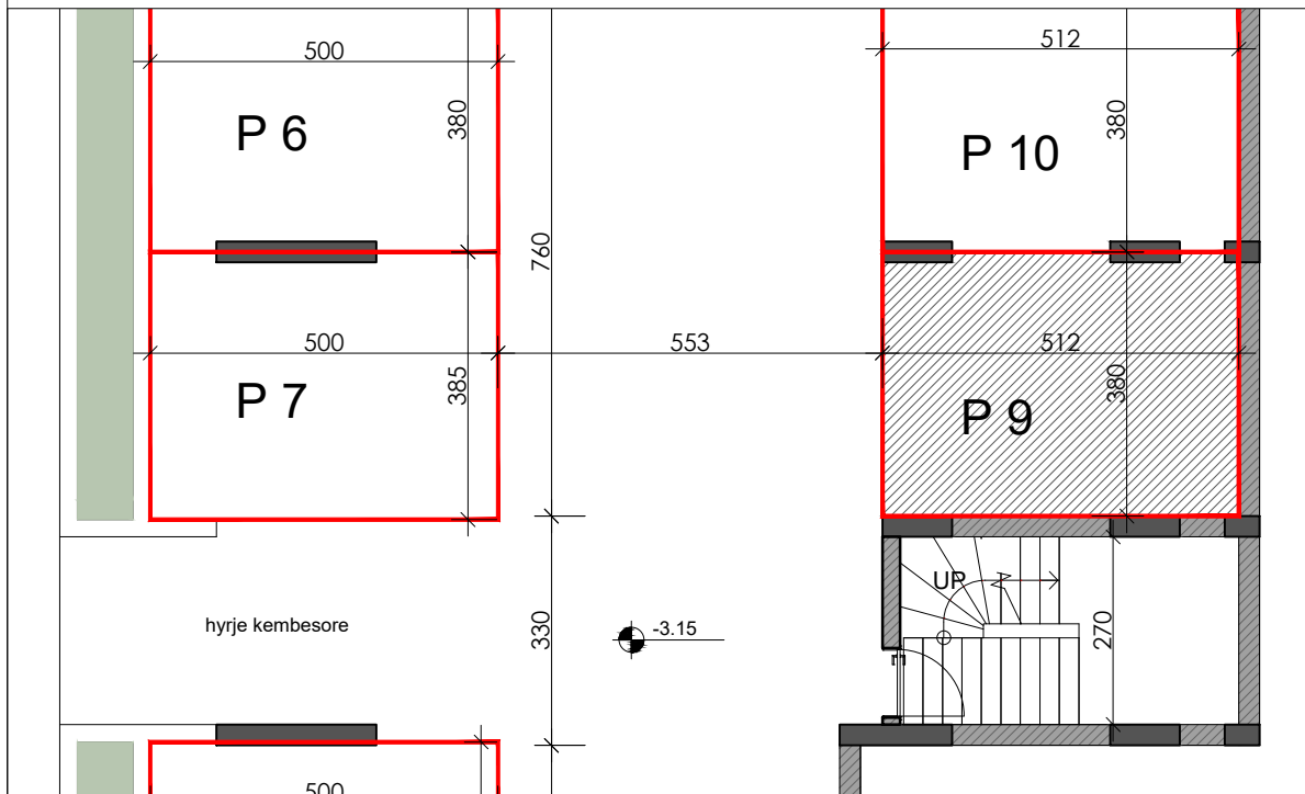
PLANIMETRIA SH 1: 100
