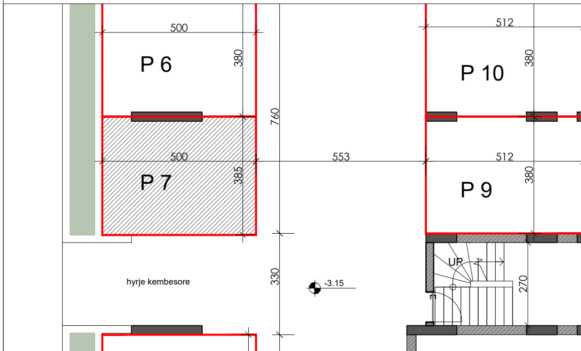
PLANIMETRIA SH 1: 100
