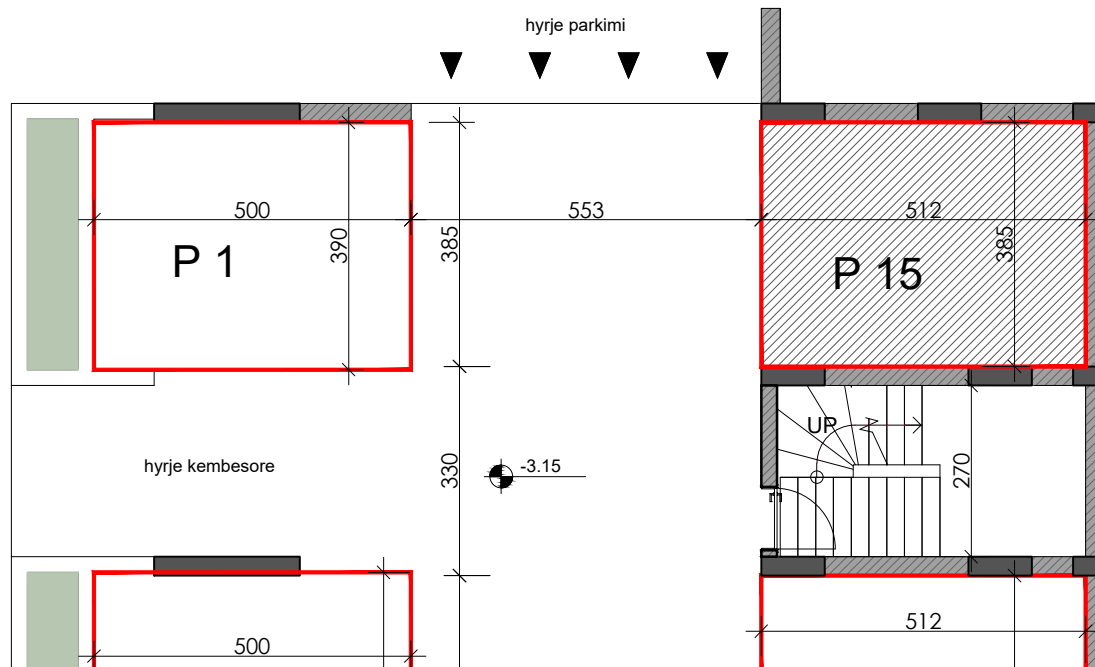
PLANIMETRIA SH 1: 100
