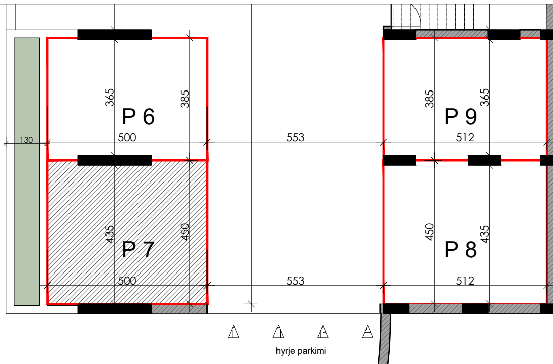
PLANIMETRIA SH 1: 100
